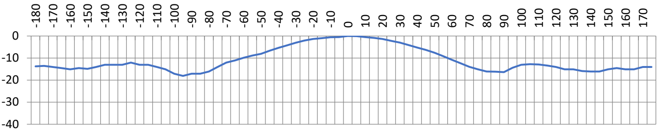
1800Mhz Planar
