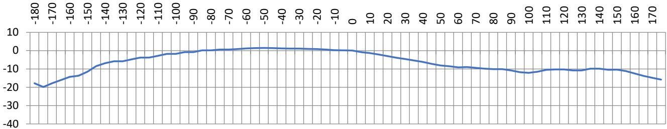
920Mhz planar
